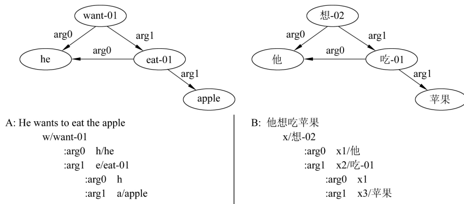
图 1 论元共享形成的图结构示例
