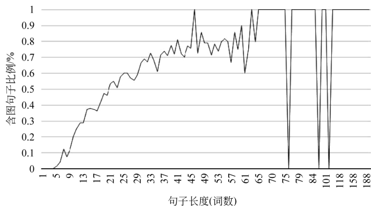
图 3 中文 CTB 语料句子长度与图结构的关系
